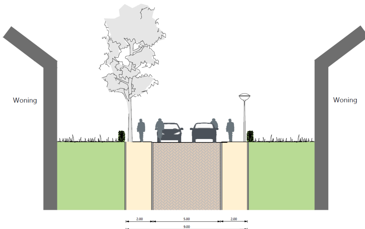
Figuur 10: Ideaalprofiel ETW, in elementverharding.
