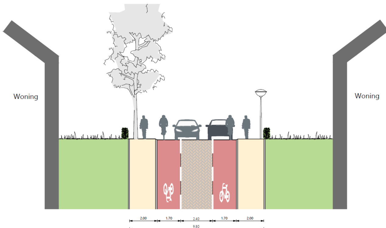
Figuur 8: Ideaalprofiel GOW30, met rode fietsstroken.
