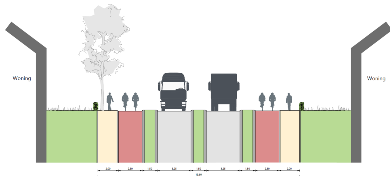
Figuur 4: Ideaalprofiel GOW50, met vrijliggende fietspaden.
