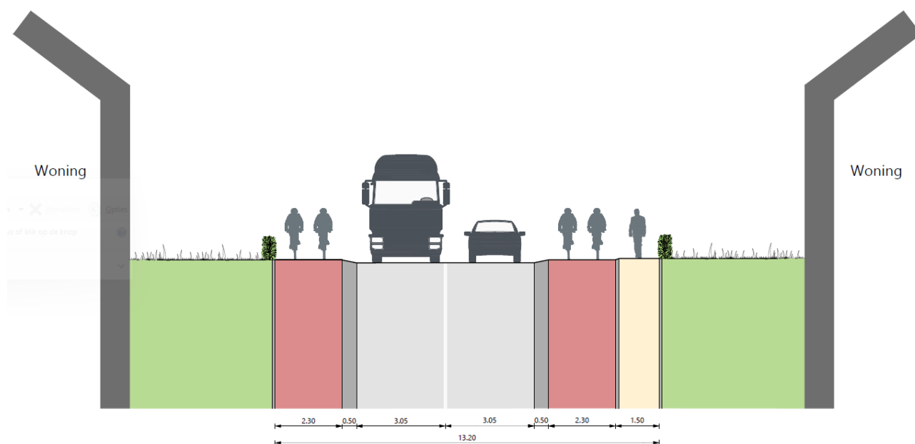
Figuur 3: Basisprofiel GOW50, met aanliggend verhoogde fietspaden.
