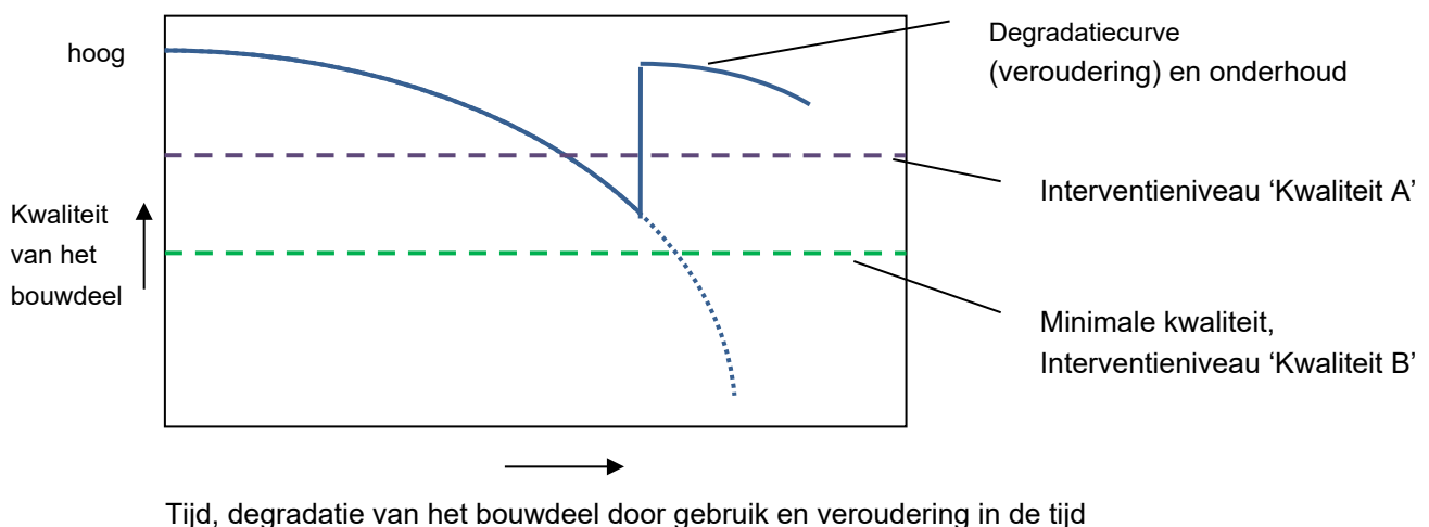
Figuur 3: Principe van toestand afhankelijk onderhoud
